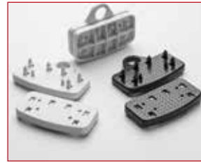
Placchette di tensionamento "Art Fix"
